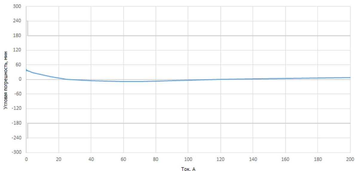
Рисунок 3.4. Фактическая угловая погрешность тока защитной обмотки.
