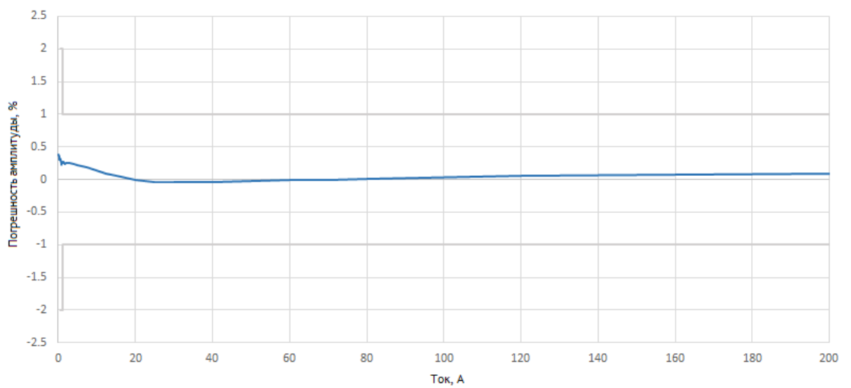
Рисунок 3.3. Фактическая погрешность измерения амплитуды тока защитной обмотки.
