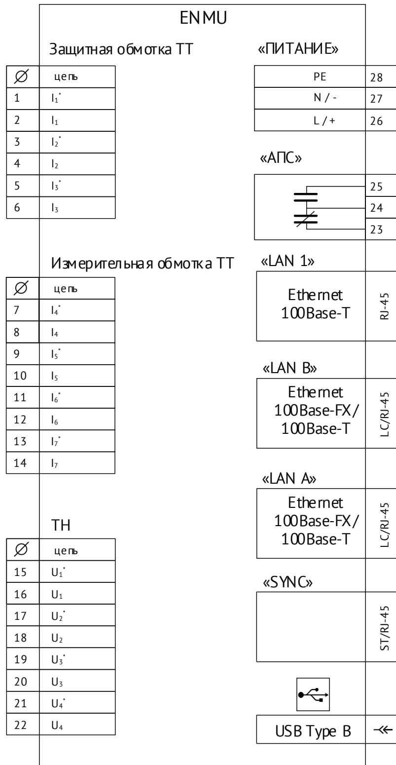
Рисунок 4.1. Измерительные входы, интерфейсы, питание.
