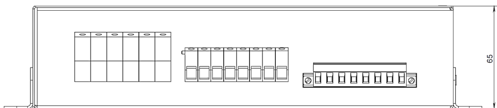
Рисунок 1.5. Габаритные размеры ENMU-X/X-X (без дополнительных интерфейсов)
